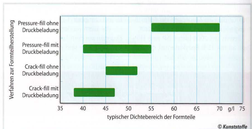
Bild 4. Arpro 5134 RE kann im Crack-fill- und Pressure-fill-Verfahren, jeweils mit oder ohne Druckbelastung, verarbeitet werden (Quelle: JSP)
