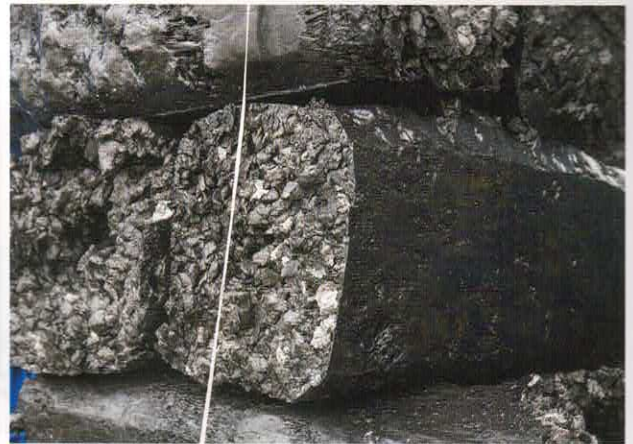
Bild 2. Die ausgemusterten Ladungsträger werden gesammelt, verdichtet und anschließend zu Granulat verarbeitet (© JSP)
